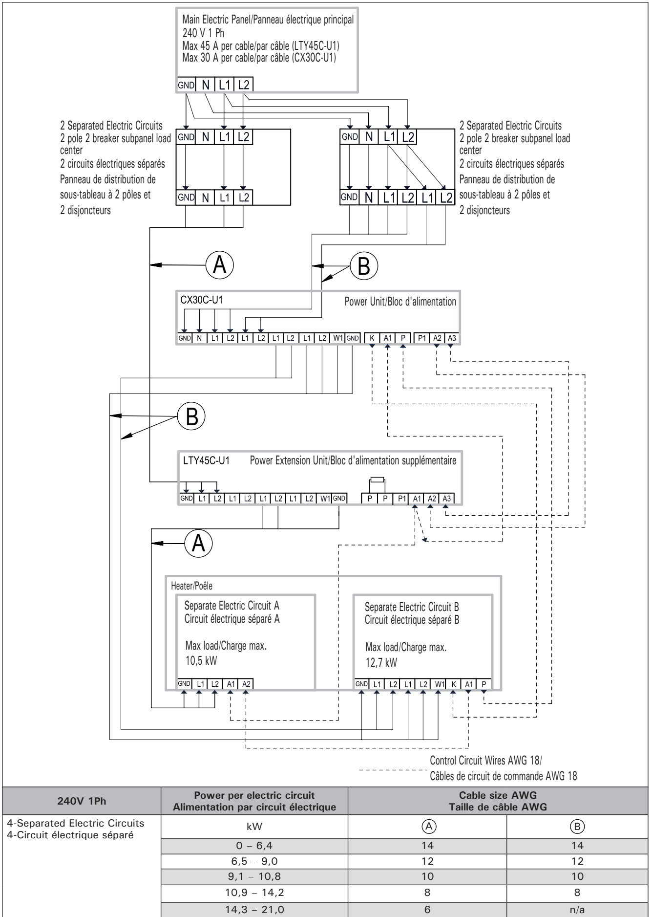
Figure 18. Connection of power extension unit LTY45C-U1 with control unit CX30C-U1 (240 V / 1Ph). Heater with one built-in steamer units and one pair of A1/A2 terminals Figure 18. Branchement du bloc d'alimentation supplémentaire LTY45-U1 au centre de contrôle CX30-U1 (240 V / 1 Ph). Poêle avec un générateur de vapeur intégré et une paire de bornes A1/A2
