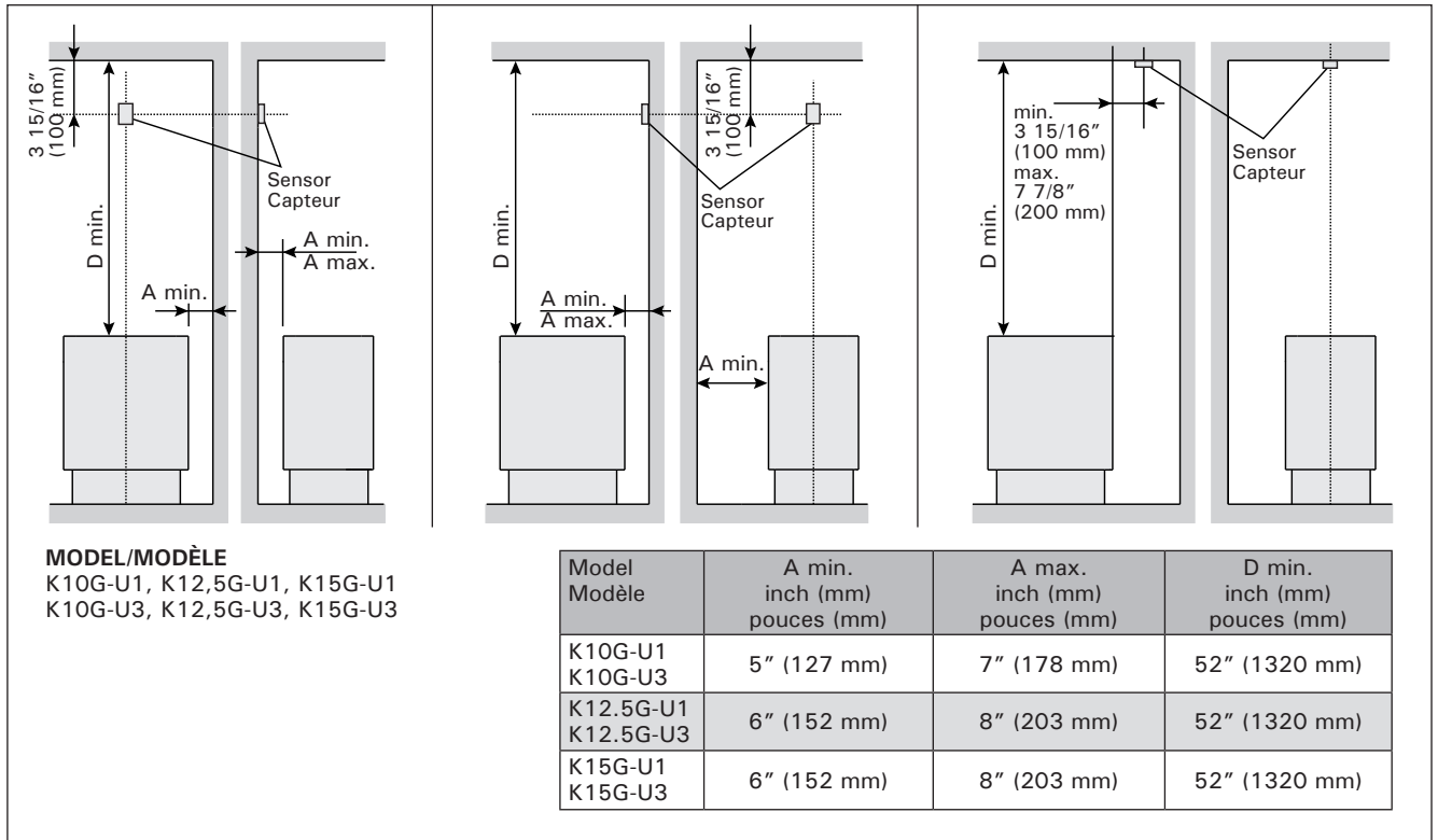
Figure 7. The place of the temperature sensor of the control unit in connection with floor-mounted heaters Figure 7. Emplacement des capteurs de température par rapport aux poêles en installation au sol
